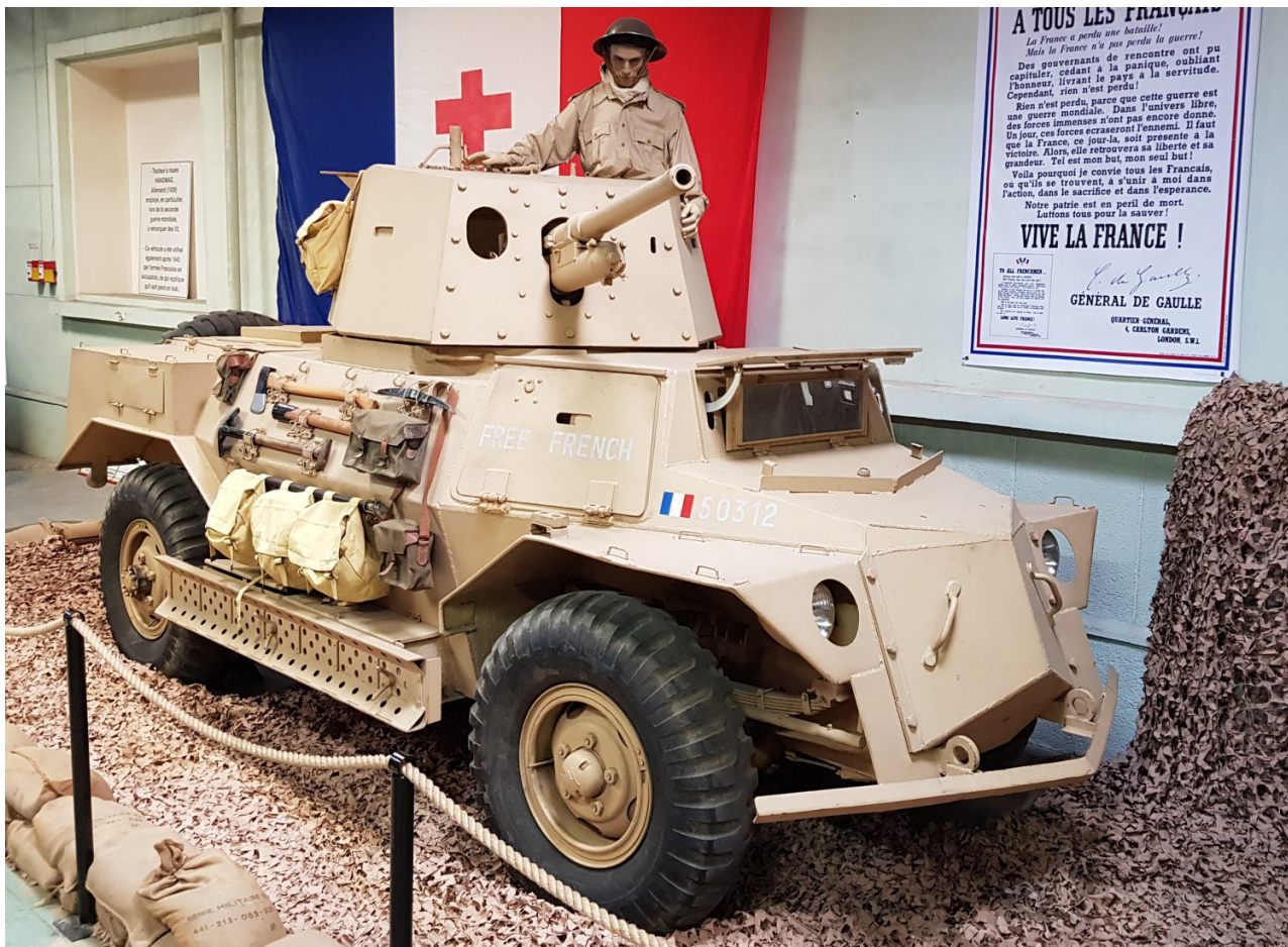
Marmon-Herrington Armoured Car Mk IV – Musée des Blindés, Saumur (France)
