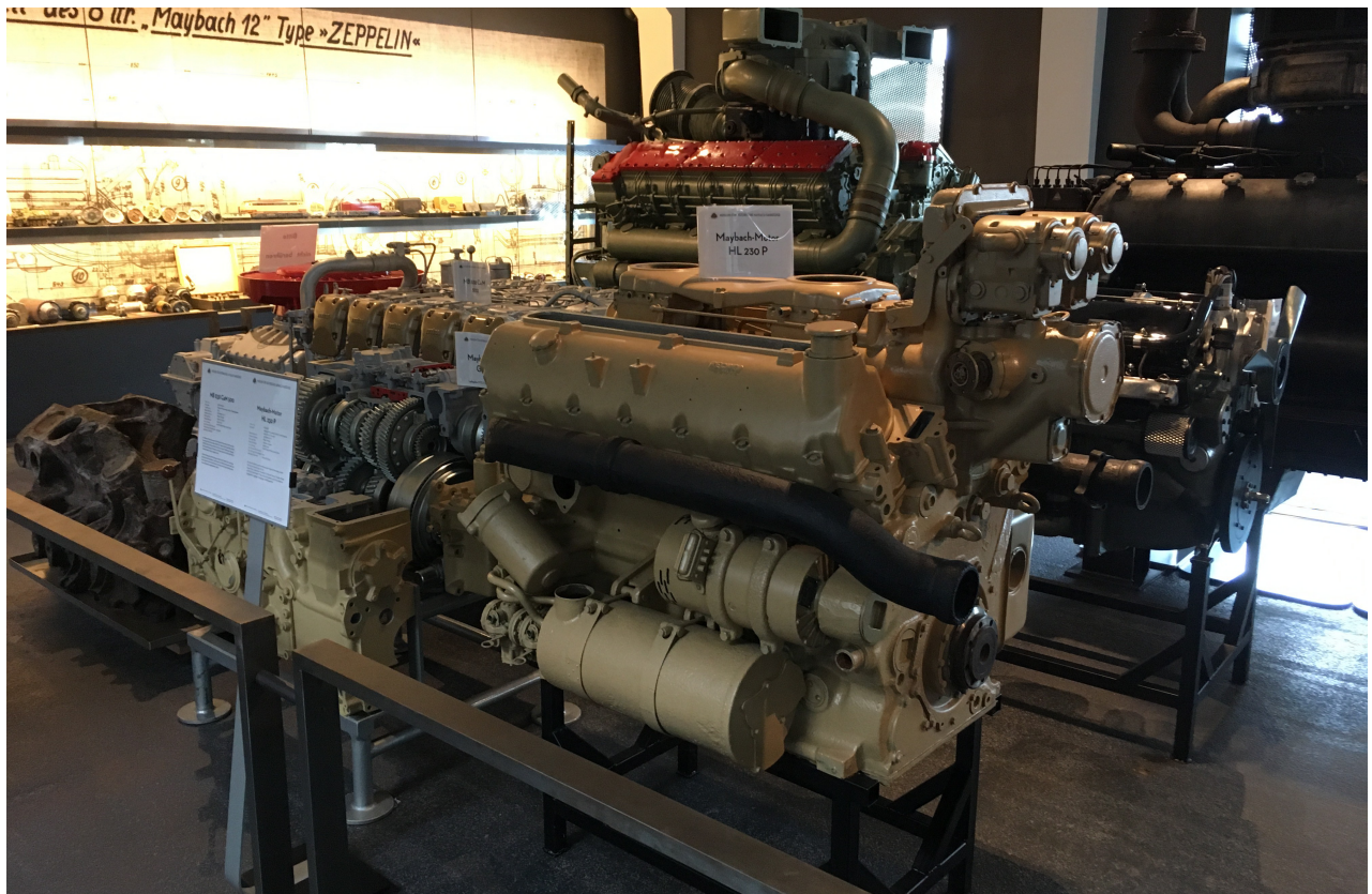
Maybach HL 230 P30 engine – Museum für historische Maybach-Fahrzeuge Oberpfalz (Germany)
