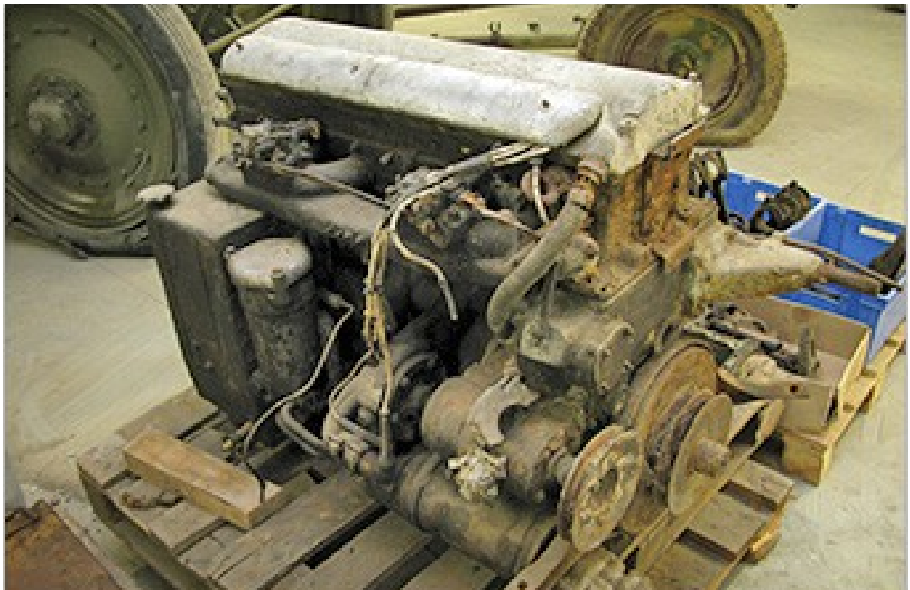
PzKpfw. II Ausf. L « Luchs » engine – ASPHM Association, La Wantzenau (France)
