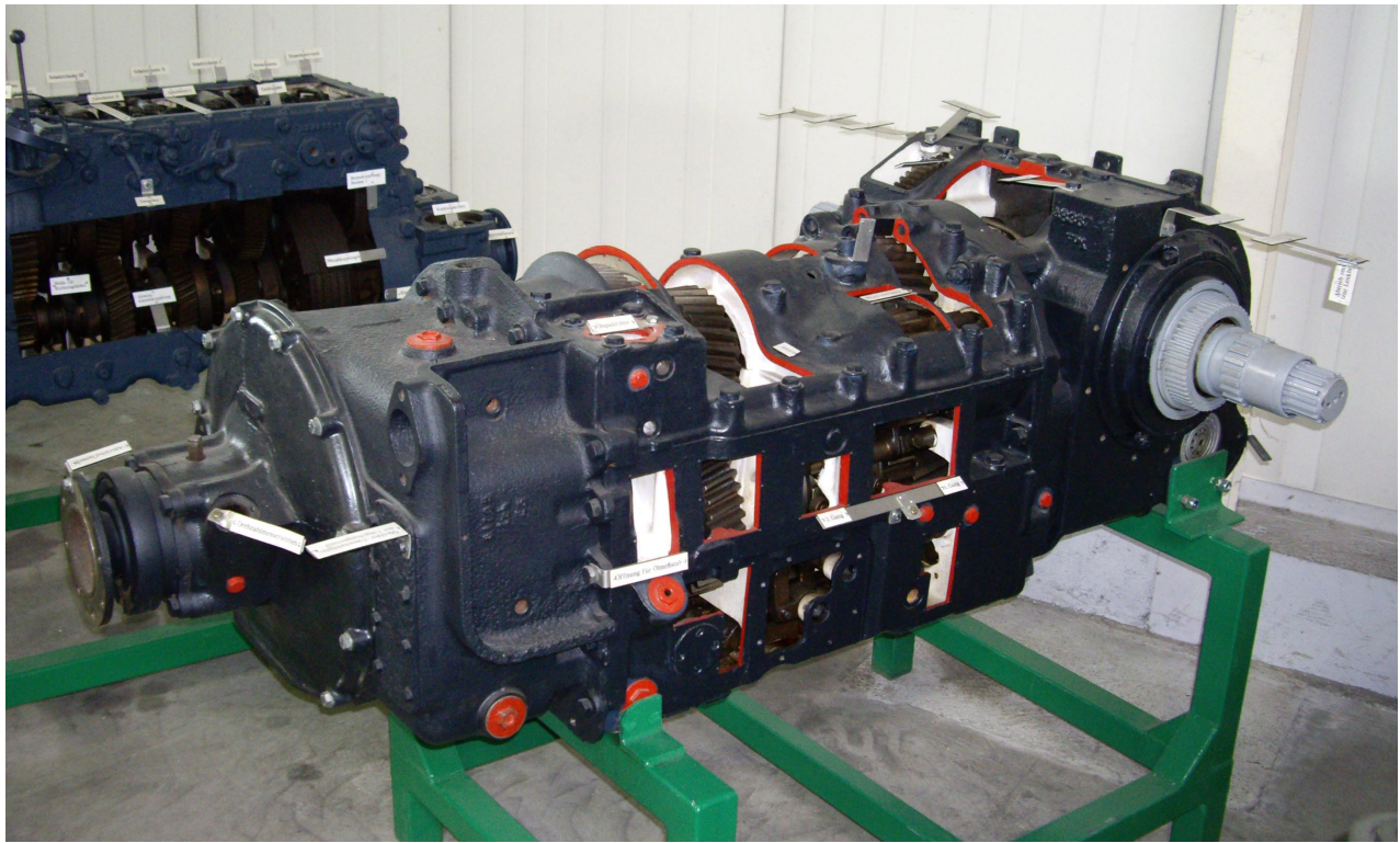
Panther gearbox – Wehrtechnische Studiensammlung Koblenz (Germany)
